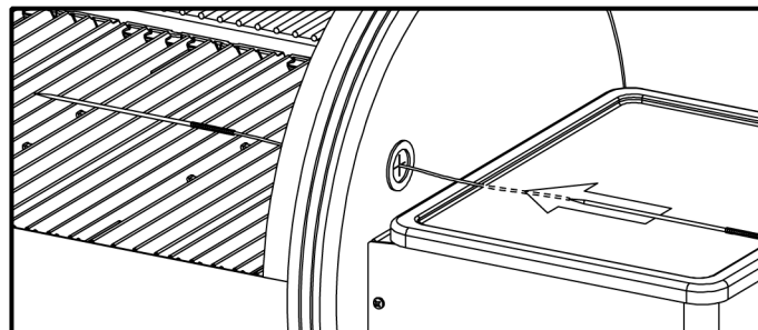
Sonde de thermomètre passant par le côté du fumoir
